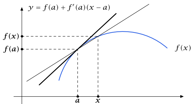
Figura 6.1 Recta tangente
