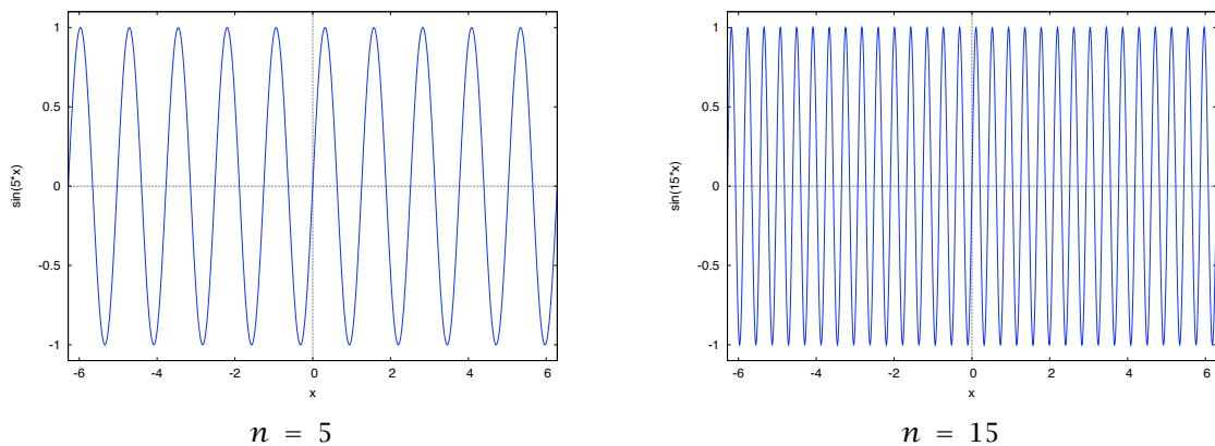
Figura 2.3 \sin(nx)
