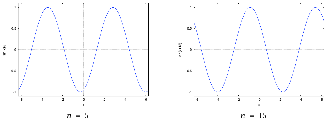
Figura 2.2 \sin(x + n)
